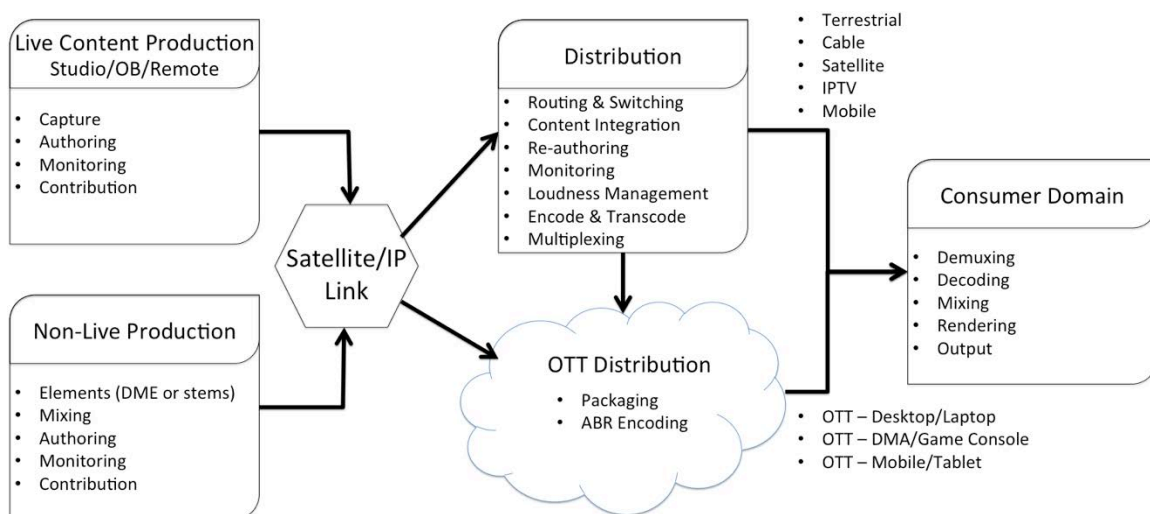
Figure 13 NGA Distribution Overview
