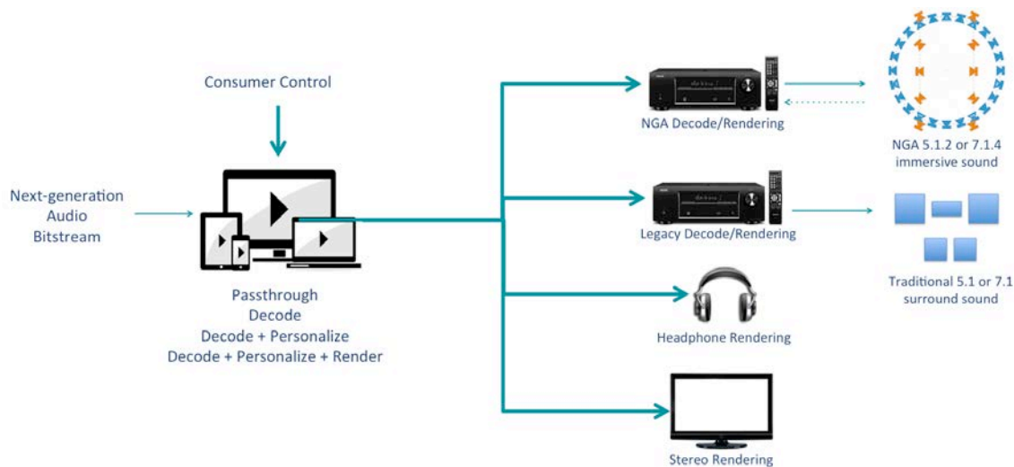
Figure 14 NGA Consumer Domain
