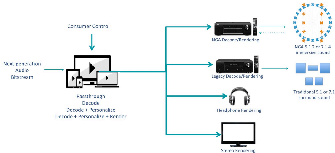
Figure 58 NGA in the consumer domain
